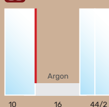
Double vitrage thermique + acoustique renforcé
