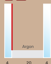
Double vitrage thermique standard
