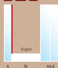
Double vitrage thermique + sécurité
