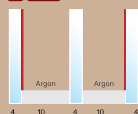
Triple vitrage thermique super renforcé
