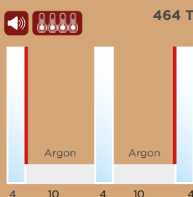
Triple vitrage thermique super renforcé
