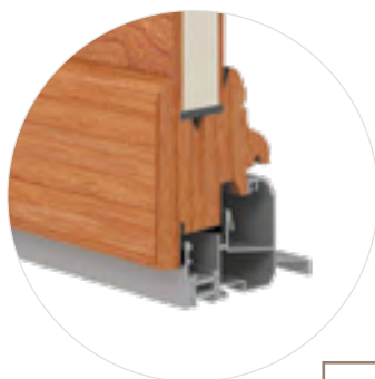
Seuil aluminium à rupture de pont thermique
